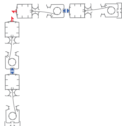
2 VANTAUX À SUIVRE ANGULAIRE
