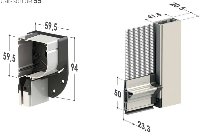
Caisson de 55
