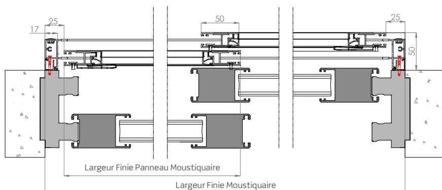
Section horizontale
