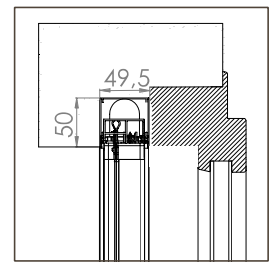
BORA ENCAS MIDI 50/50
