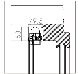
BORA ENCAS MIDI 50/35
