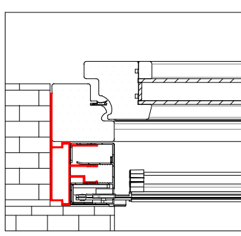
SECTION HORIZONTALE
