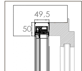
BORA TOP ENCAS SR MIDI 35
