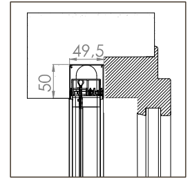
BORA ENCAS SR MIDI 20
