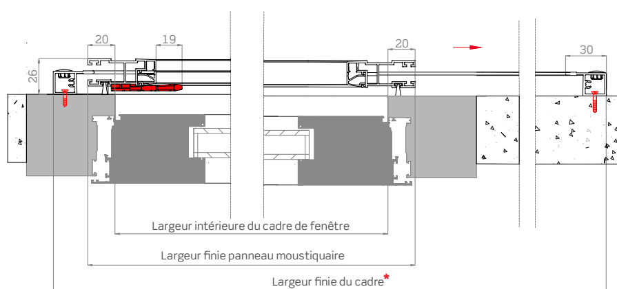
Section horizontale
