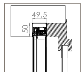
BORA TOP ENCAS MIDI 50/20
