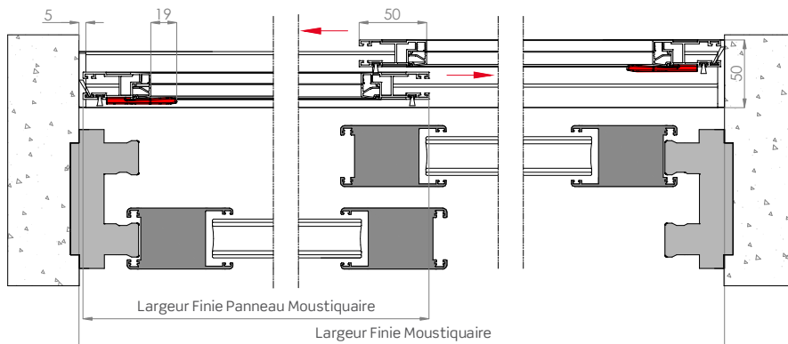
Section horizontale
