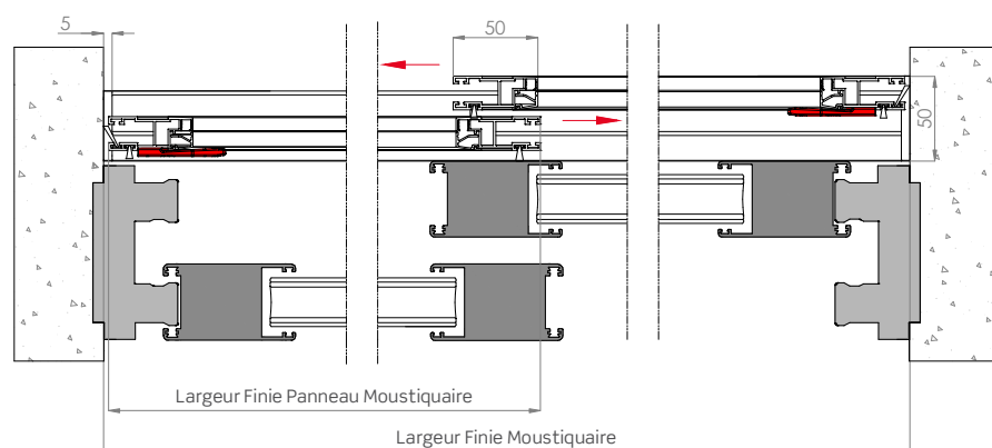
Section horizontale
