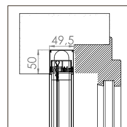
BORA ENCAS MIDI 50/20
