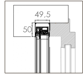
BORA TOP ENCAS SR MIDI 20
