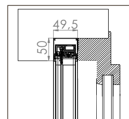
BORA TOP ENCAS MIDI 50/50
