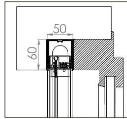
BORA TOP ENCAS SR STANDARD 20
