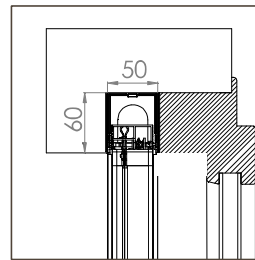
BORA ENCAS SR STANDARD 35
