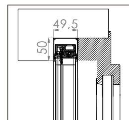
BORA TOP ENCAS MIDI 50/35
