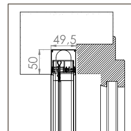
BORA ENCAS MIDI 20/20
