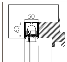
BORA TOP ENCAS SR STANDARD 50
