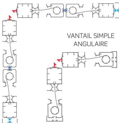
2 VANTAUX AVEC OUVERTURE BILATÉRALE ANGULAIRE
