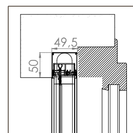
BORA ENCAS MIDI 35/35
