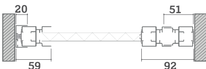
SECTION HORIZONTALE 2 VANTAUX À SUIVRE
