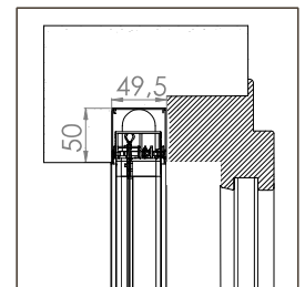
BORA ENCAS SR MIDI 50
