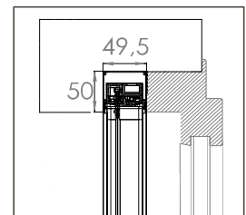
BORA TOP ENCAS SR MIDI 50
