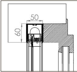
BORA TOP ANGULAIRE ENCAS 20/20 STANDARD
