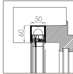
BORA ENCAS SR STANDARD 20
