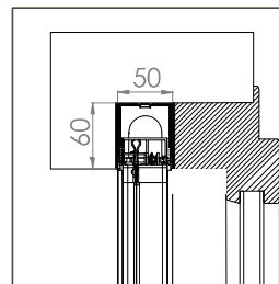
BORA ENCAS SR STANDARD 50
