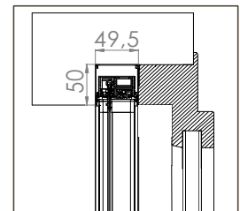
BORA TOP ENCAS MIDI 35/35
