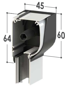
Caisson de 42
