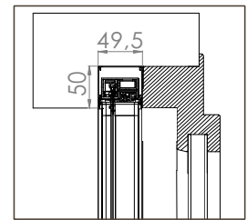
BORA TOP ENCAS MIDI 20/20
