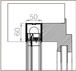
BORA TOP WINKLIG EINBAU 20/20 STANDARD
