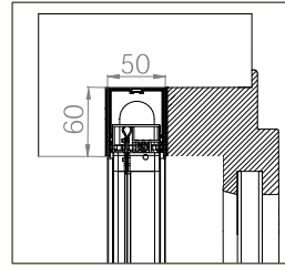
EINBAU-BORA TOP SR STANDARD 20
