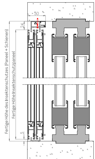
Vertikaler Abschnitt
