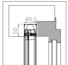
EINBAU-BORA SR MIDI 35
