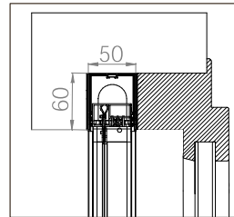
EINBAU-BORA TOP SR STANDARD 35
