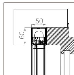
EINBAU-BORA DOPPELT STANDARD 35/35
