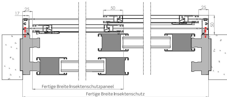
Horizontaler Abschnitt
