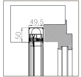
EINBAU-BORA SR MIDI 20
