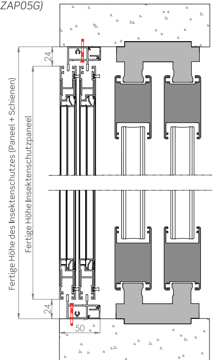
Vertikaler Abschnitt
