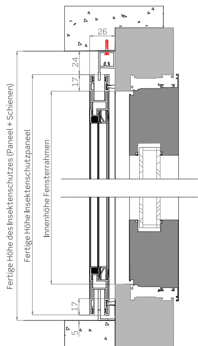
Vertikaler Abschnitt
