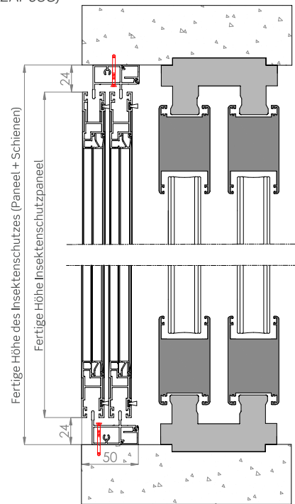
Vertikaler Abschnitt
