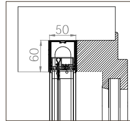
EINBAU-BORA TOP DOPPELT STANDARD 35/35
