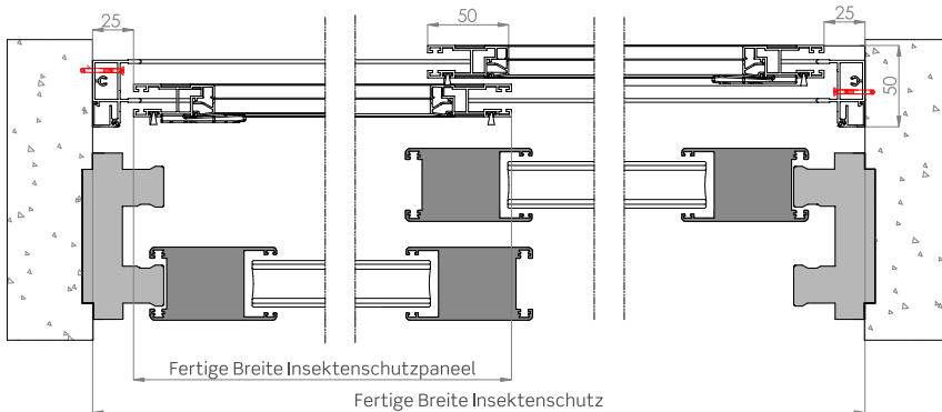
Horizontaler Abschnitt
