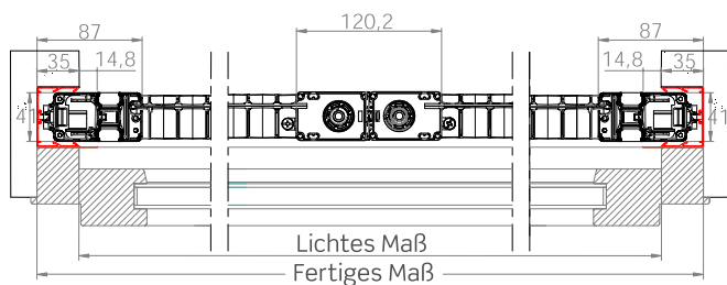
Bilaterale Öffnung
