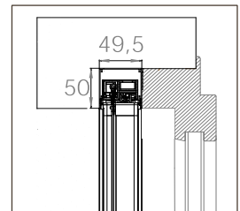
EINBAU-BORA TOP SR MIDI 50
