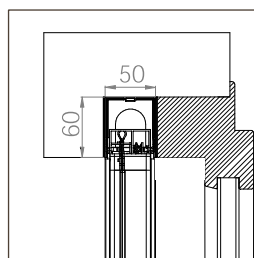
EINBAU-BORA STANDARD 35/35
