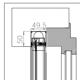
BORA EINBAU MIDI 35/35
