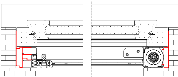
HORIZONTALER ABSCHNITT
