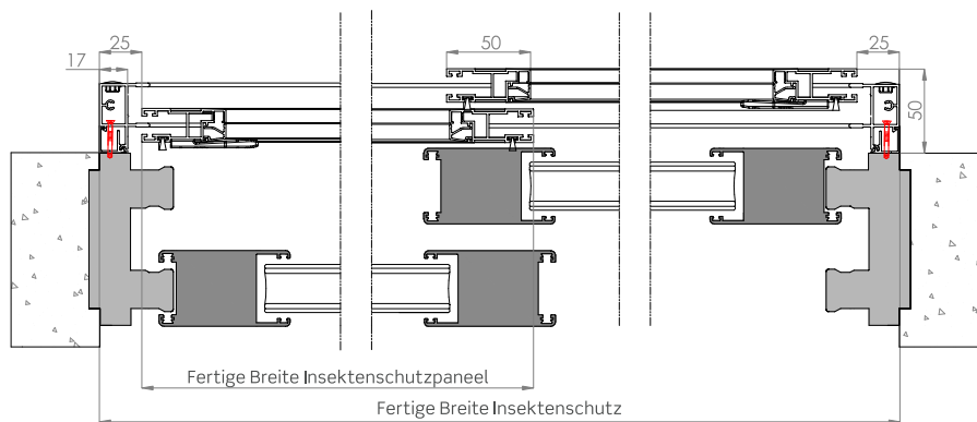
Horizontaler Abschnitt
