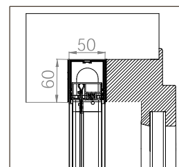
EINBAU-BORA TOP DOPPELT STANDARD 20/20
