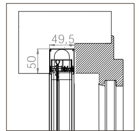
BORA EINBAU MIDI 50/50
