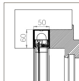
EINBAU-BORA DOPPELT STANDARD 50/50
