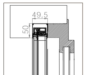
EINBAU-BORA TOP DOPPELT MIDI 20/20
