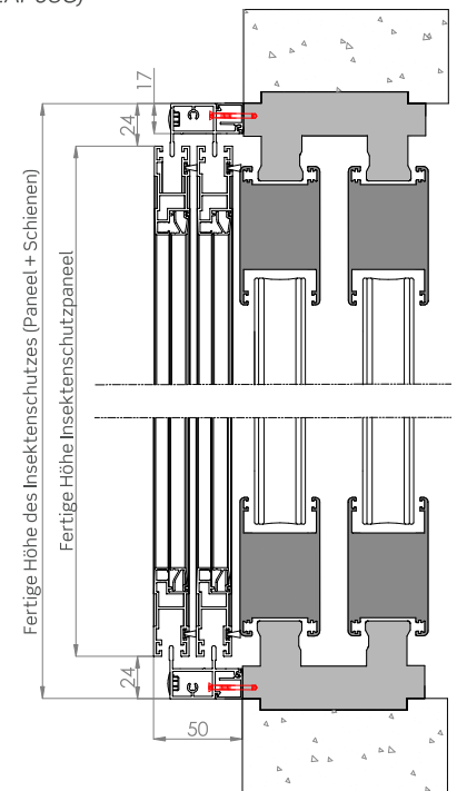
Vertikaler Abschnitt
