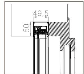
EINBAU-BORA TOP DOPPELT MIDI 35/35
