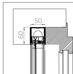
EINBAU-BORA DOPPELT STANDARD 20/20
