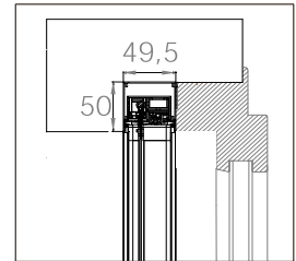
EINBAU-BORA TOP SR MIDI 35
