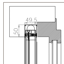
BORA EINBAU MIDI 20/20
