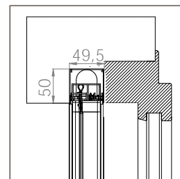
BORA EINBAU MIDI 50/20
