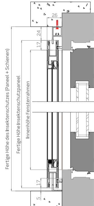
Vertikaler Abschnitt
