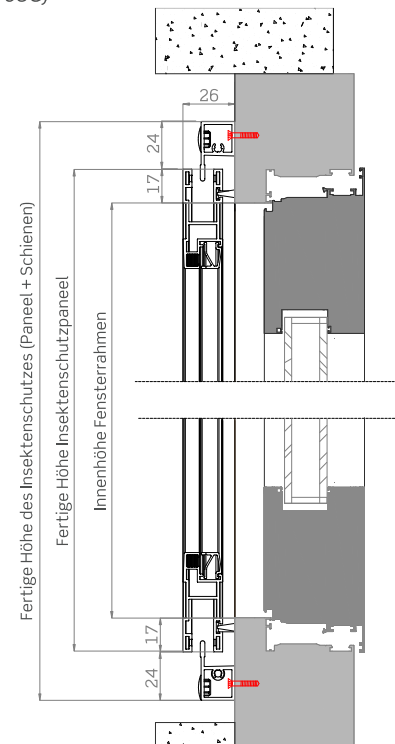
Vertikaler Abschnitt
