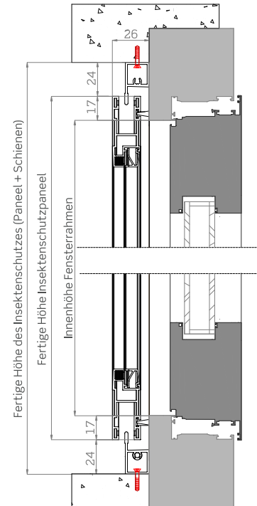
Vertikaler Abschnitt
