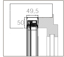
EINBAU-BORA TOP SR MIDI 20
