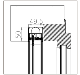
BORA EINBAU MIDI 50/35
