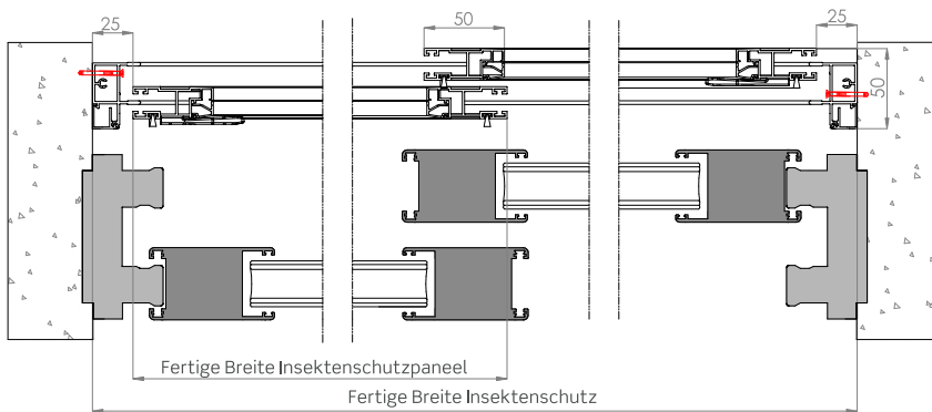
Horizontaler Abschnitt
