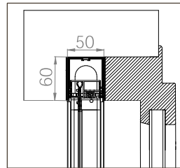
EINBAU-BORA TOP STANDARD 35/35
