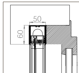
EINBAU-BORA TOP SR STANDARD 50
