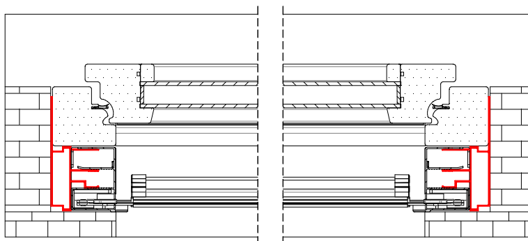
HORIZONTALER ABSCHNITT
