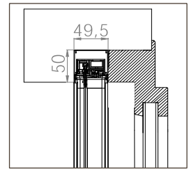
EINBAU-BORA TOP MIDI 20/20
