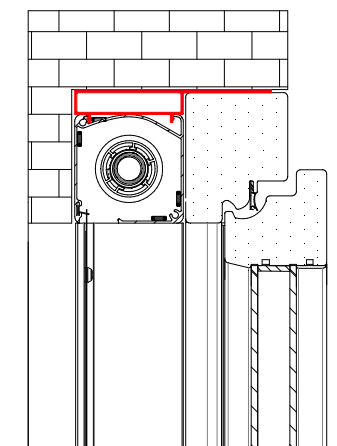
VERTIKALER ABSCHNITT
