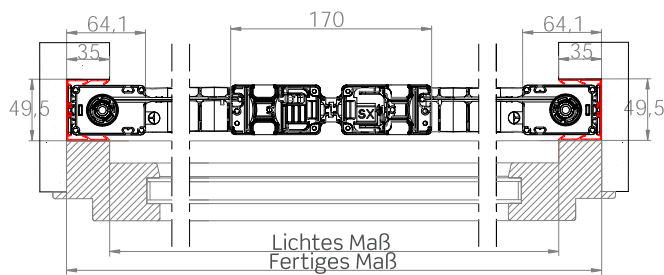
Mittige Schließung
