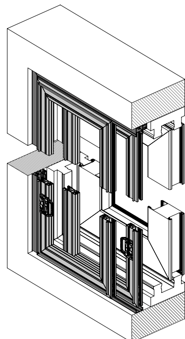
Vertikaler Abschnitt
