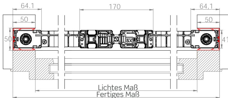
EINBAU-BORA DOPPELT STANDARD 50/50
