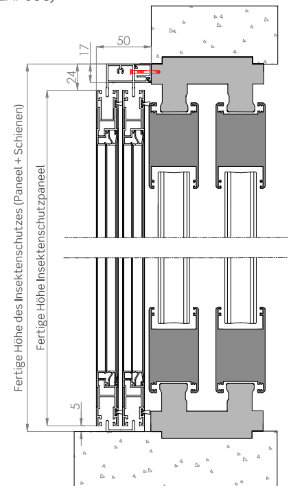
Vertikaler Abschnitt
