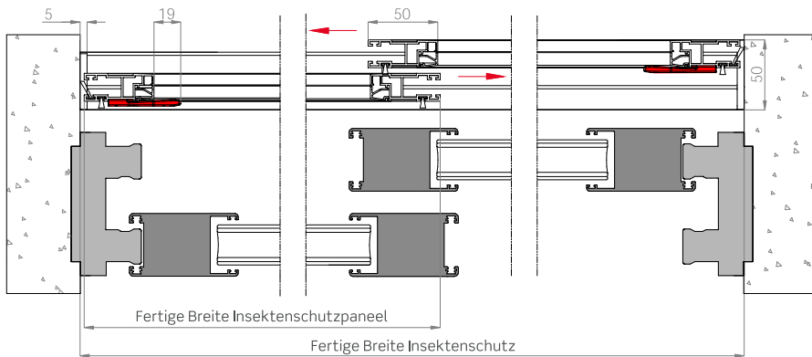
Horizontaler Abschnitt
