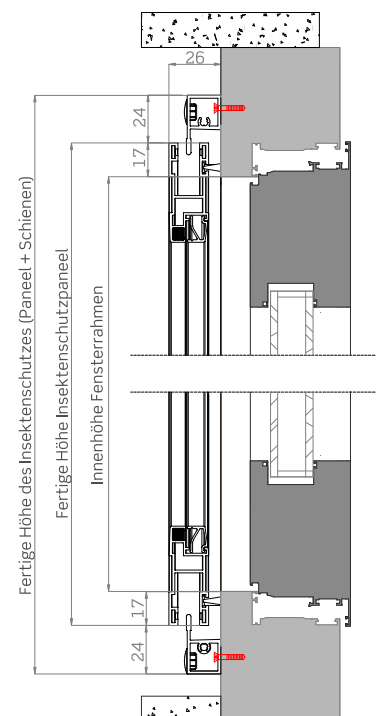
Vertikaler Abschnitt
