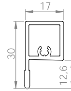
Schiene an drei Seiten (ZAP03G)
