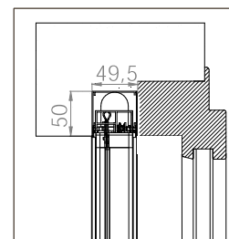
BORA EINBAU DOPPELT MIDI 35/35
