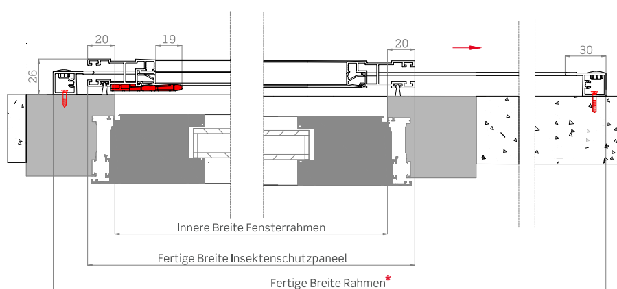
Horizontaler Abschnitt
