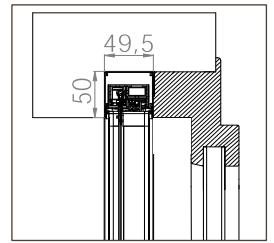
EINBAU-BORA TOP MIDI 50/50
