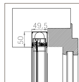
BORA EINBAU DOPPELT MIDI 50/50
