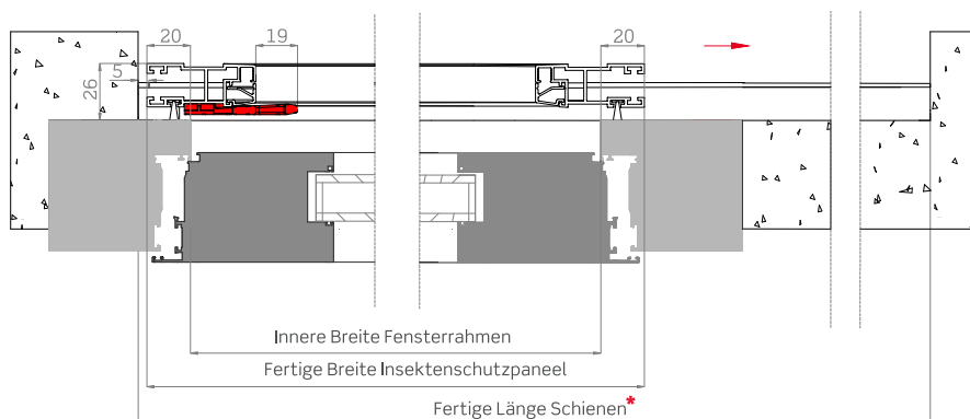
Horizontaler Abschnitt
