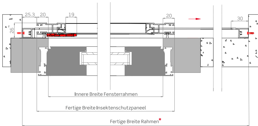
Horizontaler Abschnitt
