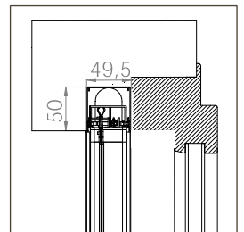
EINBAU-BORA SR MIDI 50
