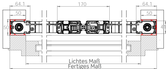
Mittige Schließung
