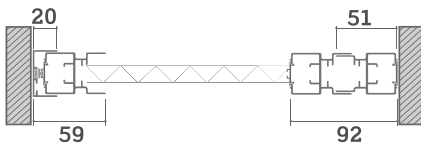
HORIZONTALER SCHNITT 2 FLÜGEL IN REIHE
