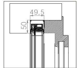
EINBAU-BORA TOP MIDI 35/35
