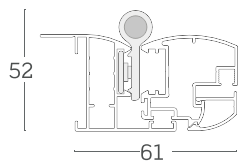
MIT RÜCKHOLFEDER
