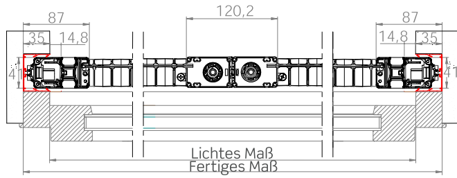
Bilaterale Öffnung
