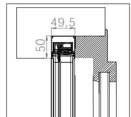
EINBAU-BORA TOP MIDI 50/20
