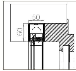
EINBAU-BORA TOP STANDARD 50/35
