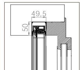
EINBAU-BORA TOP DOPPELT MIDI 50/50
