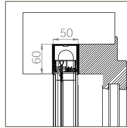
EINBAU-BORA STANDARD 50/35
