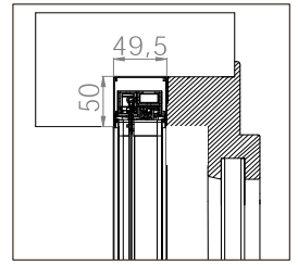
EINBAU-BORA TOP MIDI 50/35
