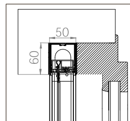
EINBAU-BORA TOP DOPPELT STANDARD 50/50
