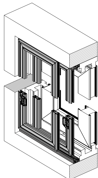
Vertikaler Abschnitt
