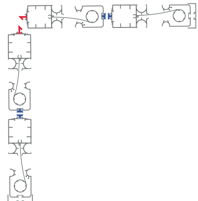
2 FLÜGEL IN REIHE UND IM WINKEL
