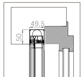
BORA EINBAU DOPPELT MIDI 20/20
