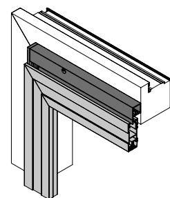
Vertikaler Abschnitt
